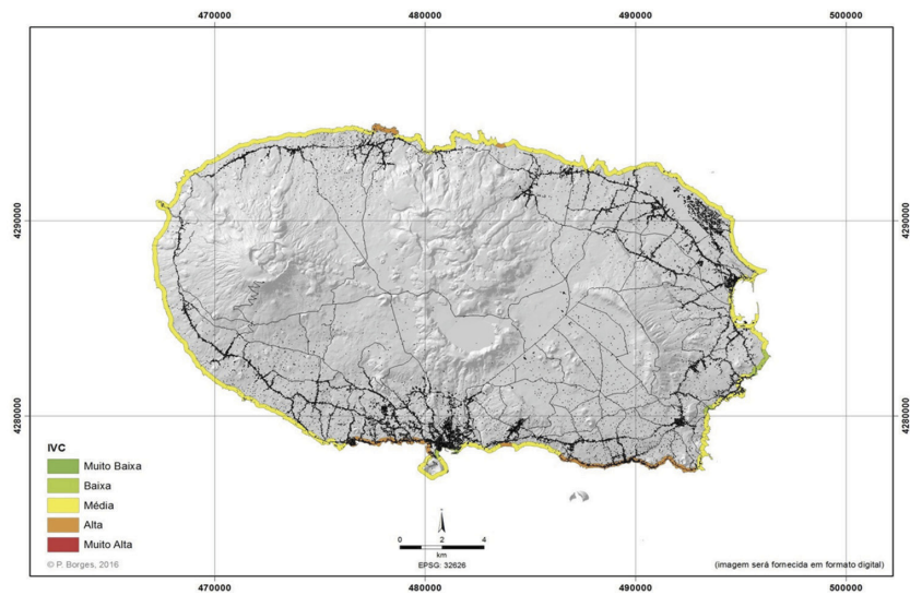
Fig. 20 — Índice de Vulnerabilidade Costeira na Ilha Terceira
